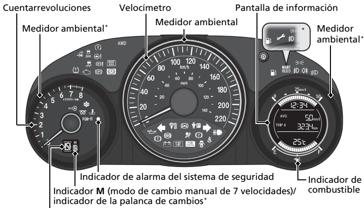
Indicador de posición de la palanca de cambios / Indicador del sistema de la caja de cambios*
